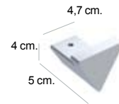
Colgador Hook ○ 44.30.01.002
